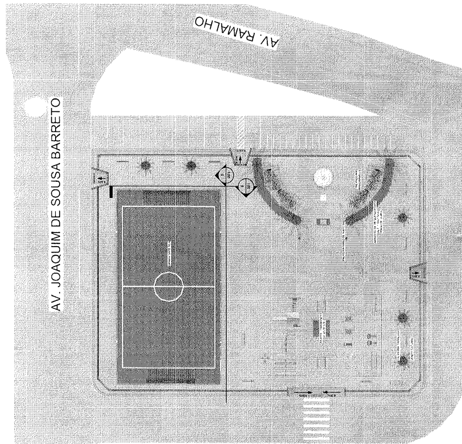
1 PLANTA BAIXA DE PAISAGISMO 1:200
