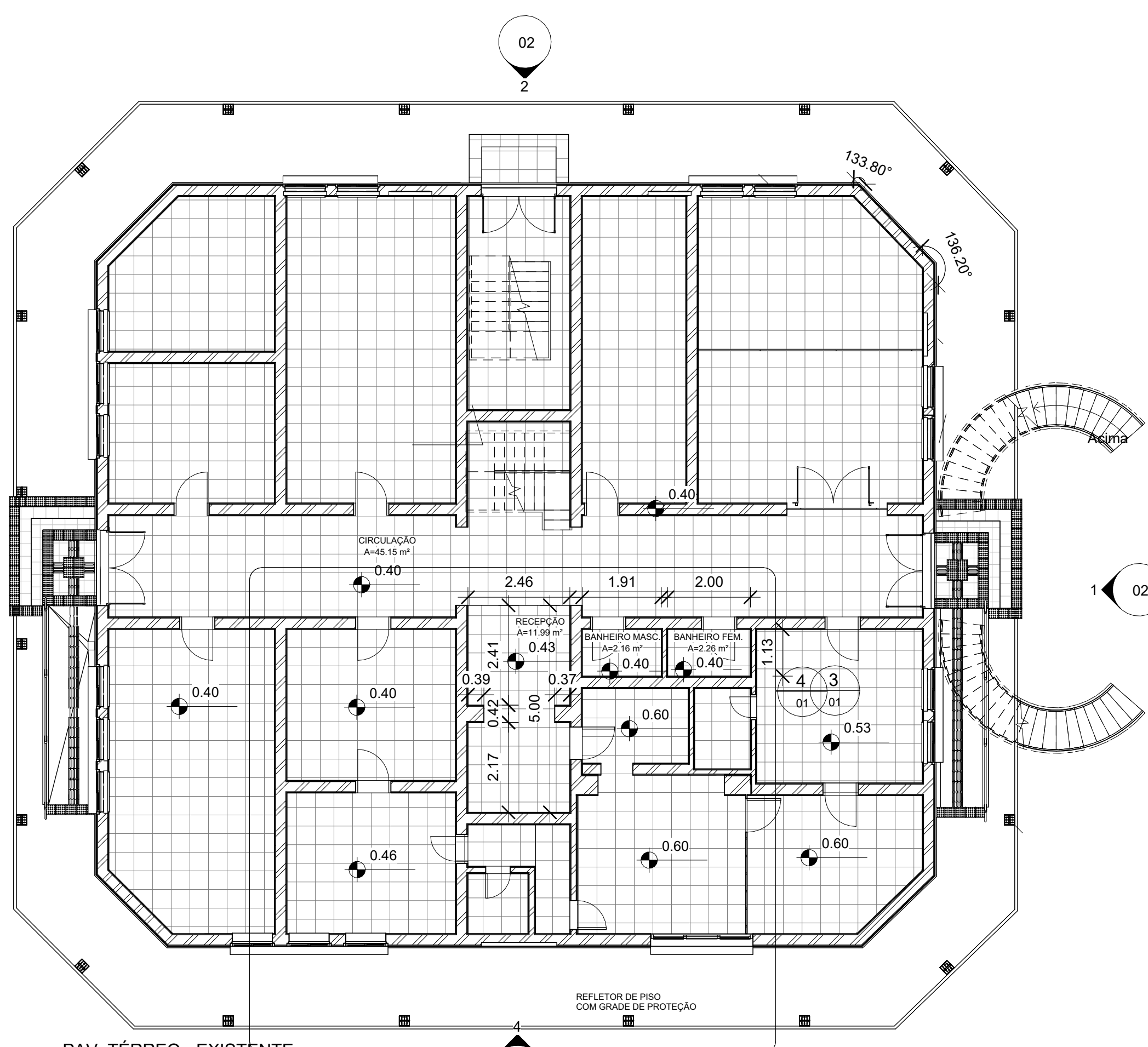
1 PAV. TÉRREO - EXISTENTE 1 : 100
