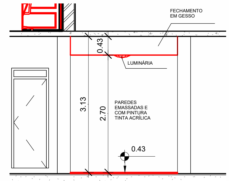
5 Corte AA 1 : 50
