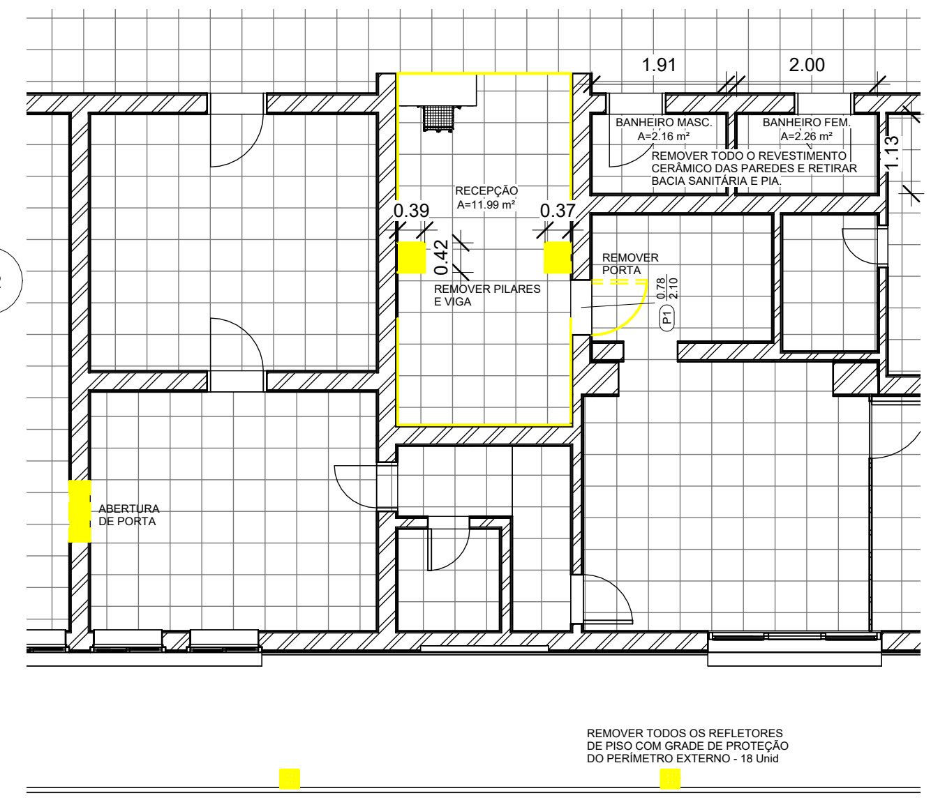
3 PAV. TÉRREO - DEMOLIR - Chamada de detalhe 1 1 : 75
