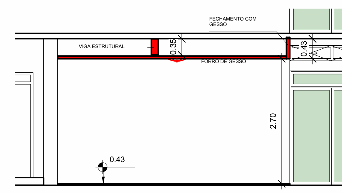
6 Corte BB 1 : 50
